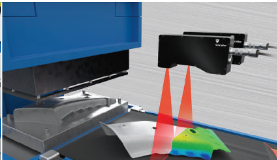
การติดตั้ง เซ็นเซอร์สองตัว ทำงานร่วมกัน ช่วยรวมโปรไฟล์เข้าด้วยกัน ใช้ในการสแกนพื้นผิวขนาดใหญ่
