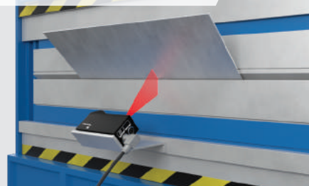
Line Profiler ใช้ในการกำหนดมุมโค้งงอสุดท้ายในเบรคแบบกด (press brake)
